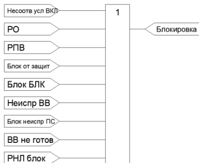
Рисунок 3.3.10 – Функциональная схема формирования сигнала блокировки РВ
