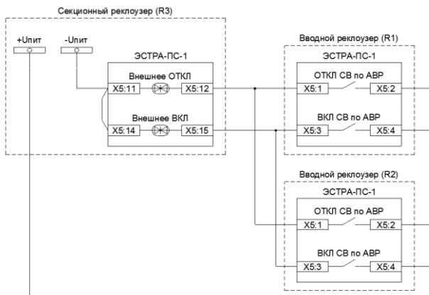
Рисунок 3.2.15 – Внешние сигналы АВР и ВНР для схемы с двумя вводными и одним секционным реклоузерами. Сигналы включения и отключения резервного ввода
