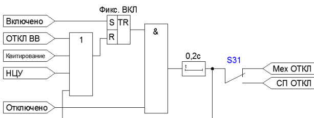
Рисунок 3.4.3 – Функциональная схема формирования сигнала отказа ВВ
