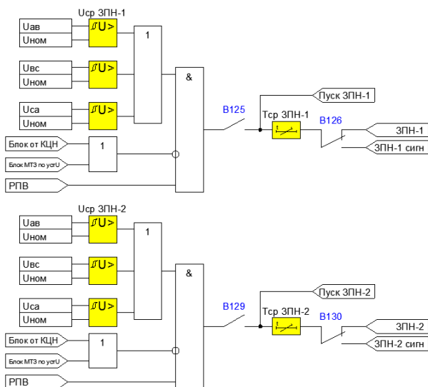
Рисунок 3.1.11 – Функциональная схема ЗПН-1 и ЗПН-2
