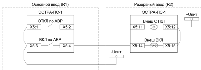
Рисунок 3.2.7 – Внешние сигналы АВР и ВНР для схемы с двумя вводными реключерами. Сигналы включения и отключения резервного ввода
