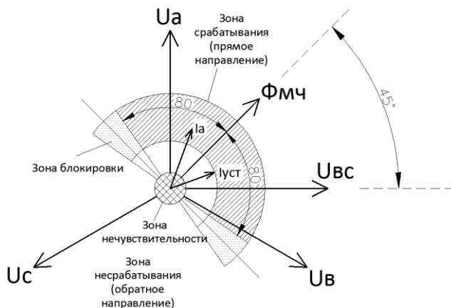
Рисунок 3.1.2 - Определение направления мощности для МТЗ
