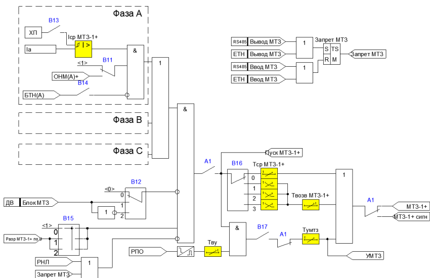
Рисунок 3.1.1 - Функциональная схема МТЗ
