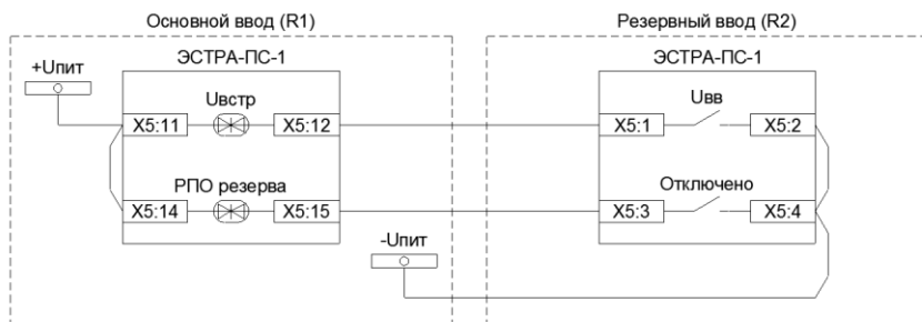
Рисунок 3.2.8 – Внешние сигналы АВР и ВНР для схемы с двумя вводными реключерами. Дополнительные сигналы контроля напряжения и положения выключателя резерва
