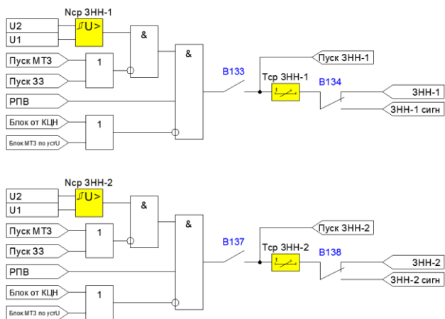
Рисунок 3.1.12 – Функциональная схема ЗНН-1 и ЗНН-2
