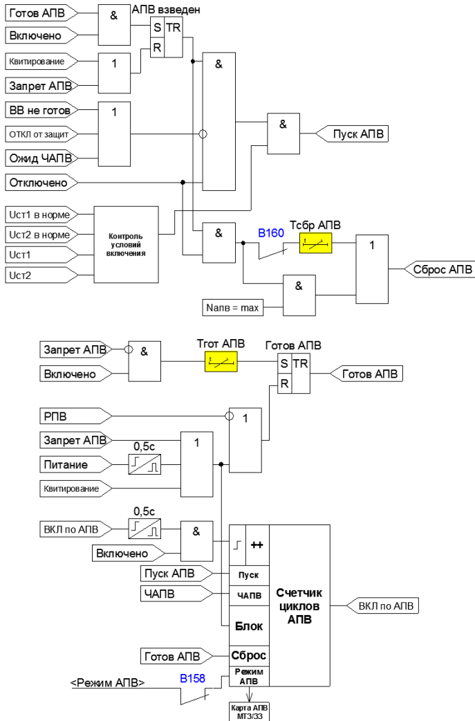
Рисунок 3.2.3 – Функциональная схема АПВ
